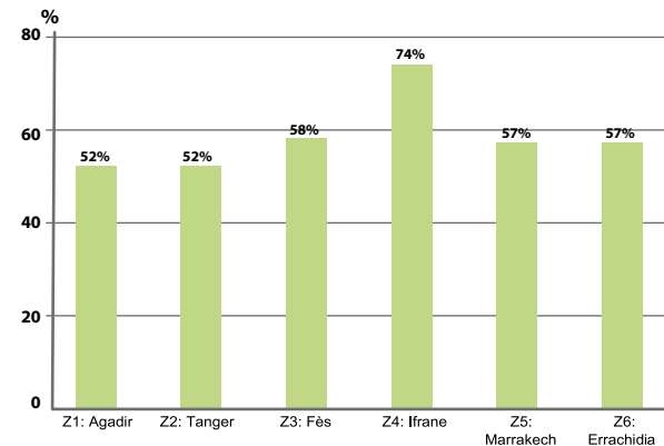
Figure 14 Impact du règlement thermique sur la réduction des besoins de chauffage et de climatisation des bâtiments administratifs au Maroc (% de réduction)
