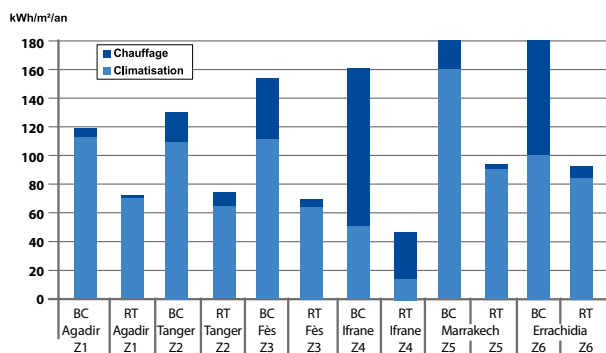
Figure 25 Comparaison cas de base (BC) et règlement thermique (RT) : bâtiment hospitalier ( T_i = 26^\circ\text{C} en été) en fonction de la zone climatique
