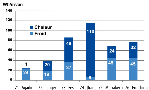
Figure 6 Gain en besoins de chaleur et en froid selon les zones climatiques
