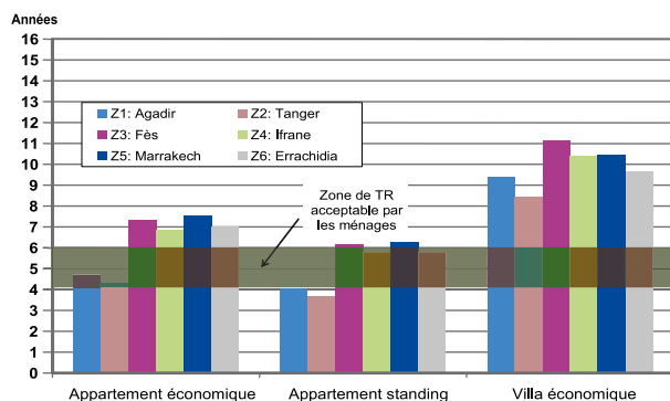
Figure 12 Temps de retour pour le consommateur final selon la zone et la catégorie d'habitat
