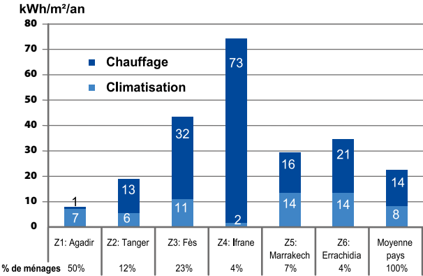
Figure 8 Economie d'énergie finale pour le chauffage et la climatisation selon les zones climatiques
