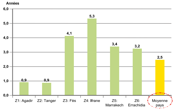
Figure 18 Temps de retour pour le consommateur final selon la zone climatique : bâtiments administratifs.
