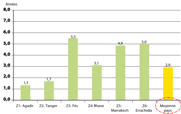
Figure 35 Temps de retour pour le consommateur final selon la zone climatique : établissements hôteliers
