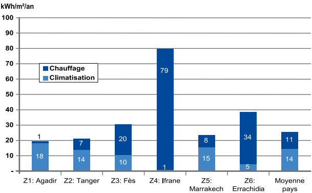
Figure 32 Economie d'énergie finale pour le chauffage et la climatisation selon les zones climatiques : établissements hôteliers
