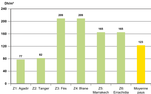
Figure 23 Surcoût d’investissement moyen engendré par le règlement thermique selon les zones climatiques : établissements scolaires
