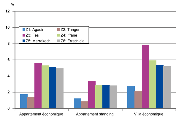
Figure 11 Pourcentage de surcoût d'investissement dû au RTCM selon la catégorie du logement et la région
