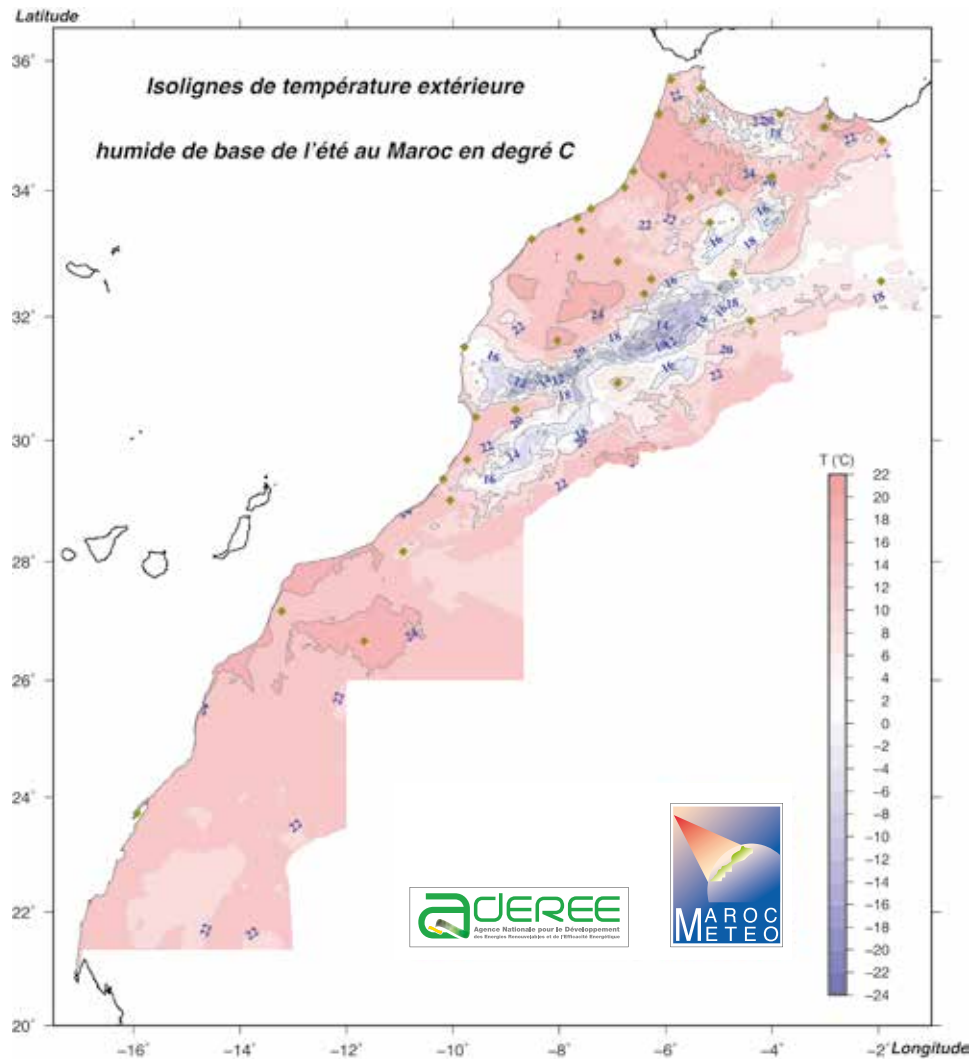
Figure 37 Carte des iso-températures extérieures humides de base de l'été calculées en se basant sur la correction par rapport à l'altitude.
