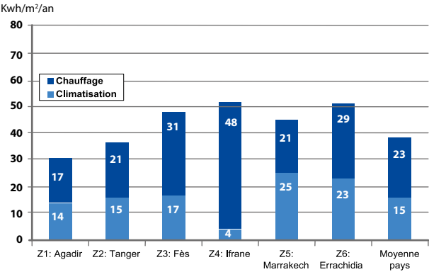
Figure 15 Economie d'énergie finale pour le chauffage et la climatisation selon les zones climatiques : administration
