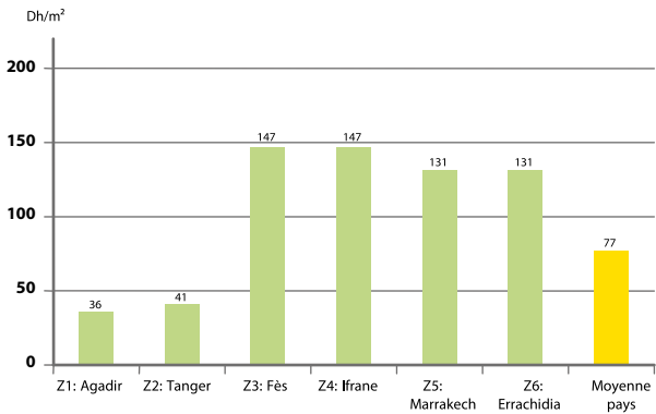
Figure 34 Surcoût d'investissement moyen engendré par le règlement thermique selon les zones climatiques : établissements hôteliers
