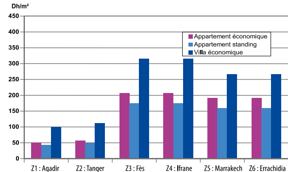
Figure 10 Surcoût d'investissement engendré par le RTCM selon les zones climatiques
