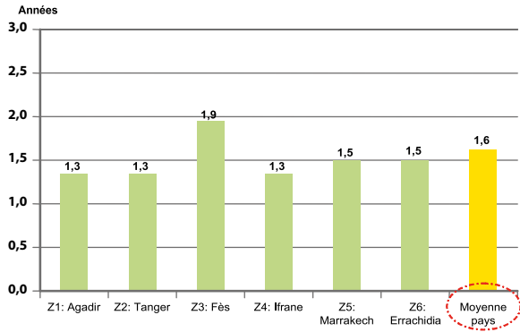
Figure 30 Temps de retour pour le consommateur final selon la zone climatique : bâtiments hospitaliers
