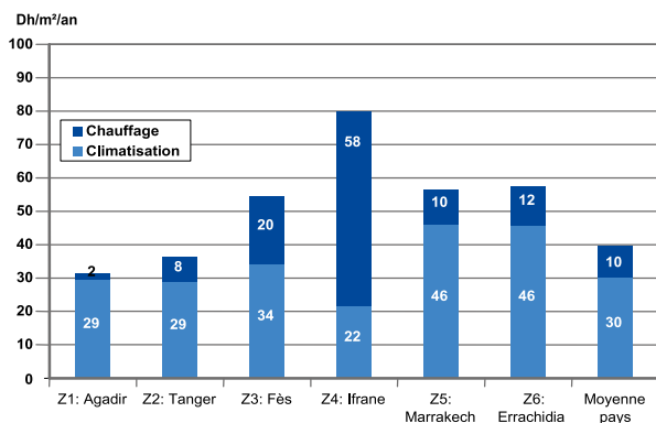
Figure 28 Gains sur facture énergétique pour le consommateur selon les zones climatiques : bâtiments hospitaliers
