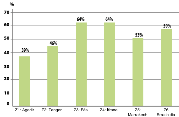
Figure 7 Impact du règlement thermique sur la réduction des besoins de chauffage et de climatisation des bâtiments résidentiels ( T_i = 26^{\circ}\text{C} en été) au Maroc (% de réduction)
