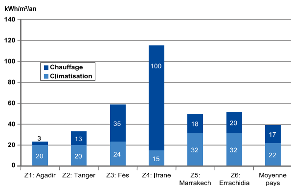
Figure 27 Economie d'énergie finale pour le chauffage et la climatisation selon les zones climatiques : bâtiments hospitaliers
