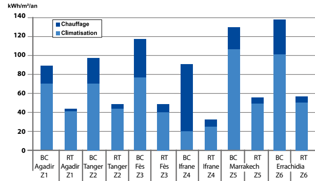
Figure 13 Comparaison cas de base (BC) et règlement thermique (RT) : bâtiment administratif ( T_i = 26^\circ\text{C} en été) en fonction de la zone climatique
