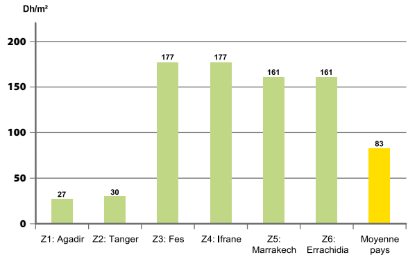
Figure 17 Surcoût d'investissement moyen engendré par le règlement thermique selon les zones climatiques : bâtiments administratifs.
