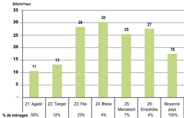
Figure 9 Gains sur la facture énergétique pour le consommateur selon les zones climatiques
