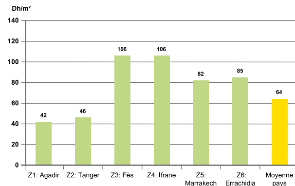
Figure 29 Surcoût d'investissement moyen engendré par le règlement thermique selon les zones climatiques : bâtiments hospitaliers
