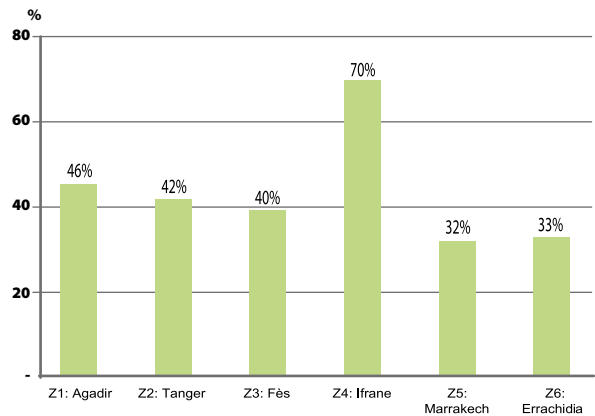
Figure 20 Impact du règlement thermique sur la réduction des besoins de chauffage et de climatisation des bâtiments scolaires au Maroc (% de réduction)
