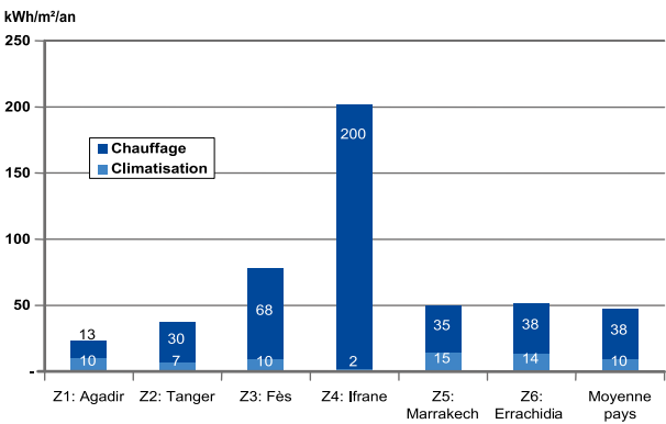
Figure 21 Economie d'énergie finale pour le chauffage et la climatisation selon les zones climatiques : établissements scolaires
