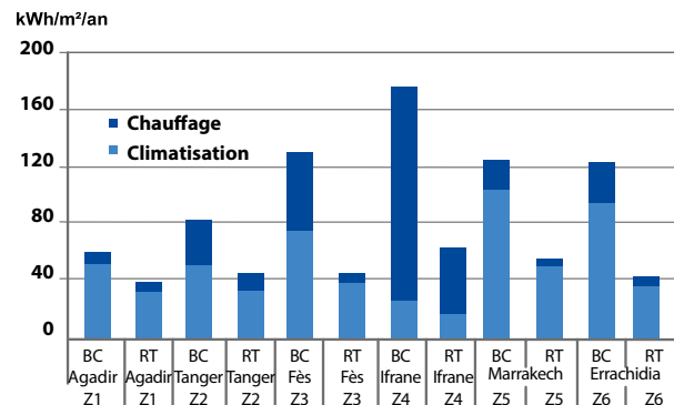
Figure 5 Comparaison cas de base et règlement thermique Bâtiment résidentiel ( T_i = 26^\circ\text{C} en été) en fonction de la zone climatique
