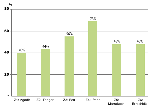
Figure 26 Impact du règlement thermique sur la réduction des besoins de chauffage et de climatisation des bâtiments hospitaliers au Maroc (% de réduction)
