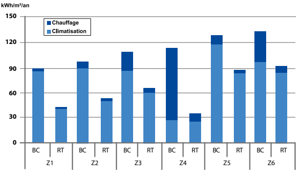
Figure 31 Comparaison cas de base et règlement thermique-établissements hôteliers (Ti = 26°C en été) en fonction de la zone climatique
