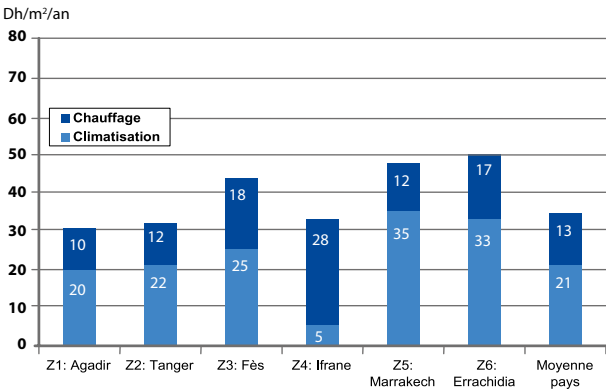
Figure 16 Gains sur la facture énergétique pour le consommateur selon les zones : bâtiments administratifs.
