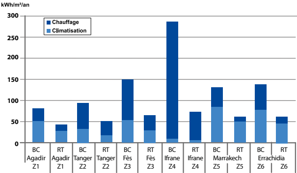
Figure 19 Comparaison cas de base et règlement thermique- bâtiments scolaires (Ti = 26°C en été) en fonction de la zone climatique
