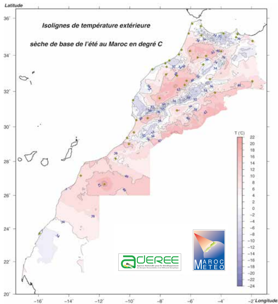
Figure 36 Carte des iso-températures extérieures sèches de base de l'été calculées en se basant sur la correction par rapport à l'altitude.
