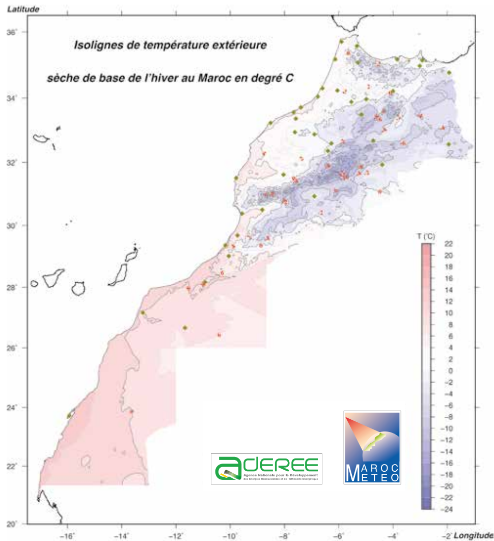
Figure 38 Carte des iso-températures extérieures sèches de base de l'hiver calculées en se basant sur la correction par rapport à l'altitude.
